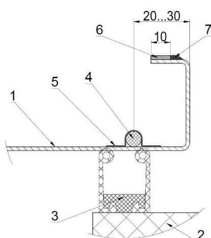
Рисунок 15. Узел крепления ПЭНа на раме
