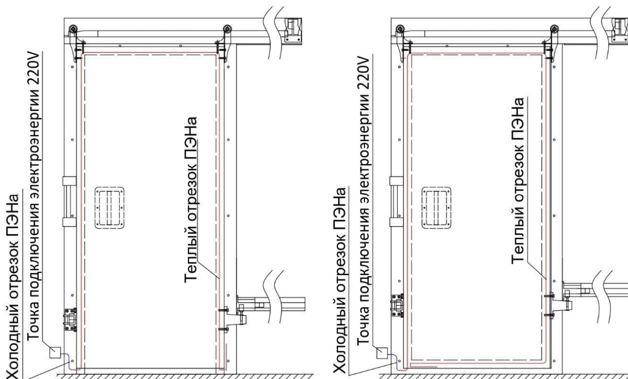
Рисунок 14: Схема расположения провода ПЭН в накладной раме Слева — исполнение рамы без порога; справа — с порогом
