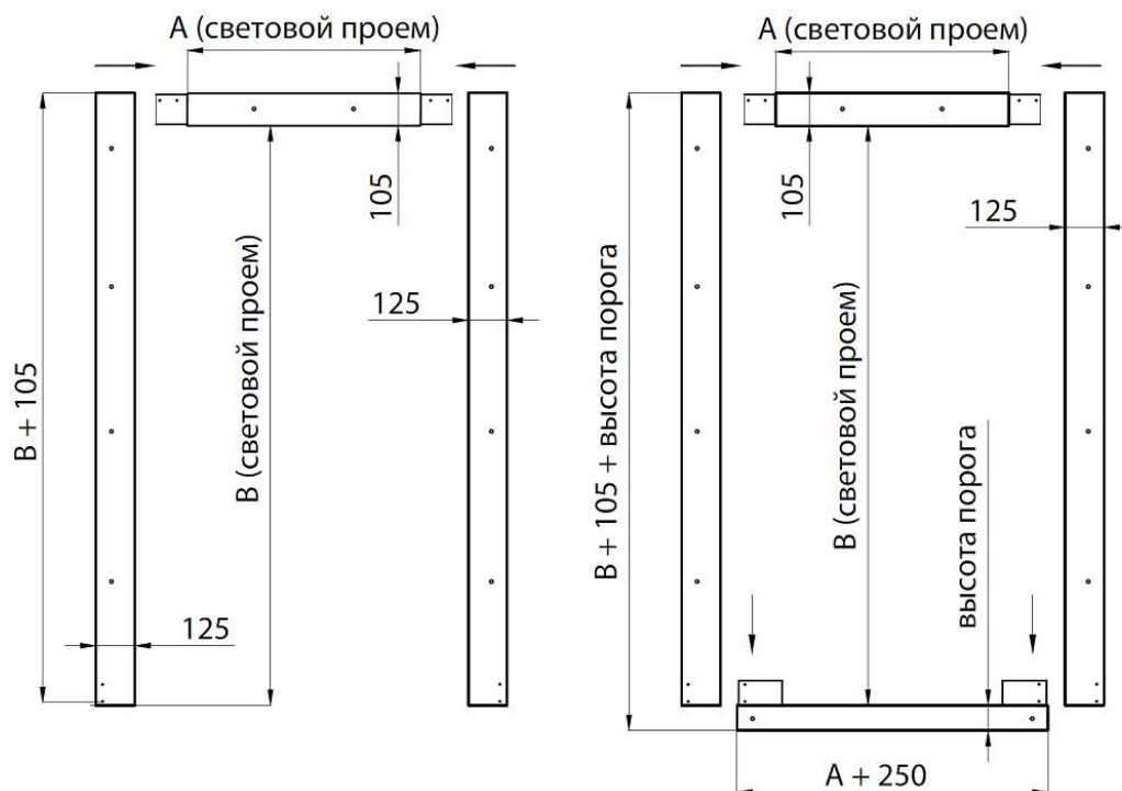
Рисунок 4. Металлическая накладная рама для дверей ОД «Оптима». Слева – без порога, справа – с порогом
